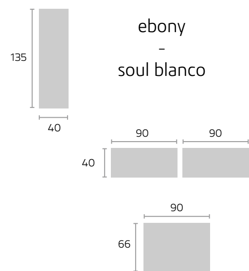
detalle aparador
